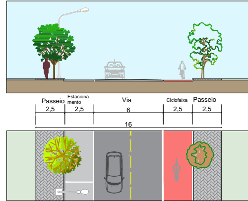
VIA LOCAL COM CICLOFAIXA
