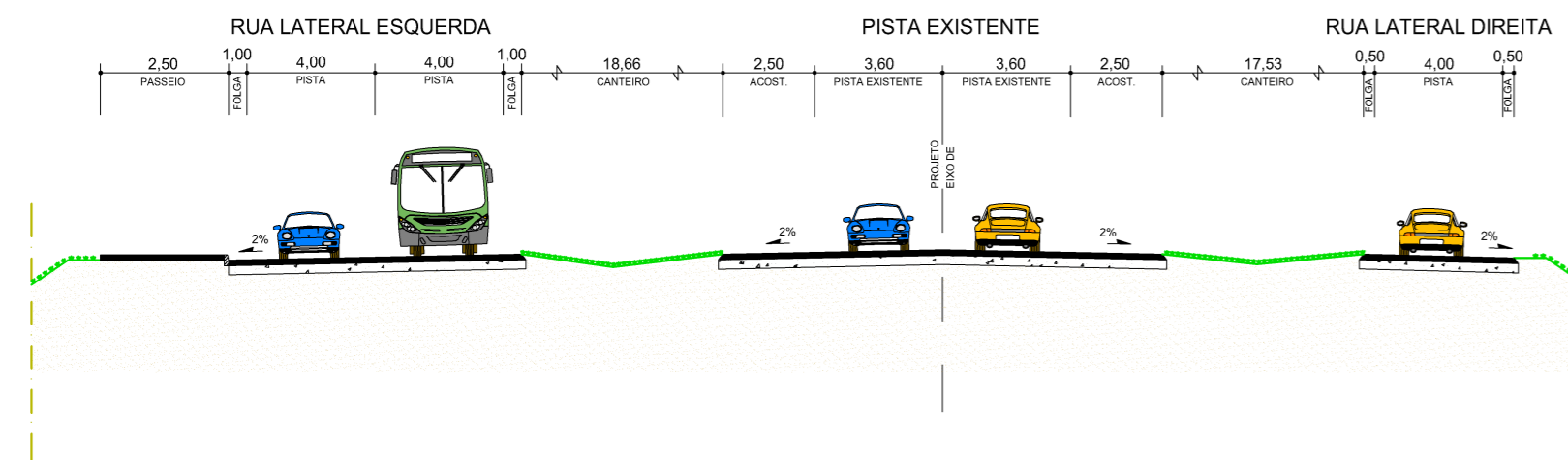
SEÇÃO TRANSVERSAL - CORTE A A' ESC: 1/200
