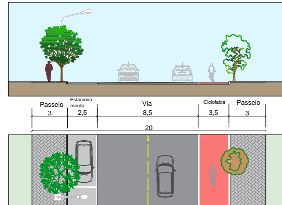
VIA COLETORA COM CICLOFAIXA
