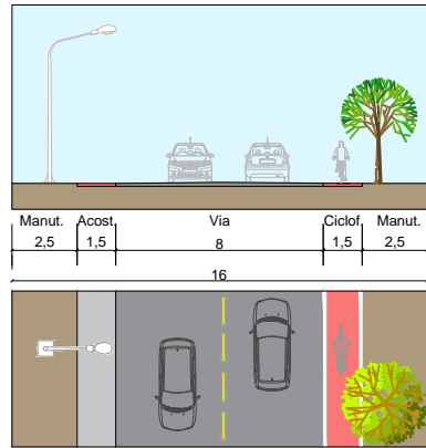
ESTRADA RURAL COM CICLOFAIXA
